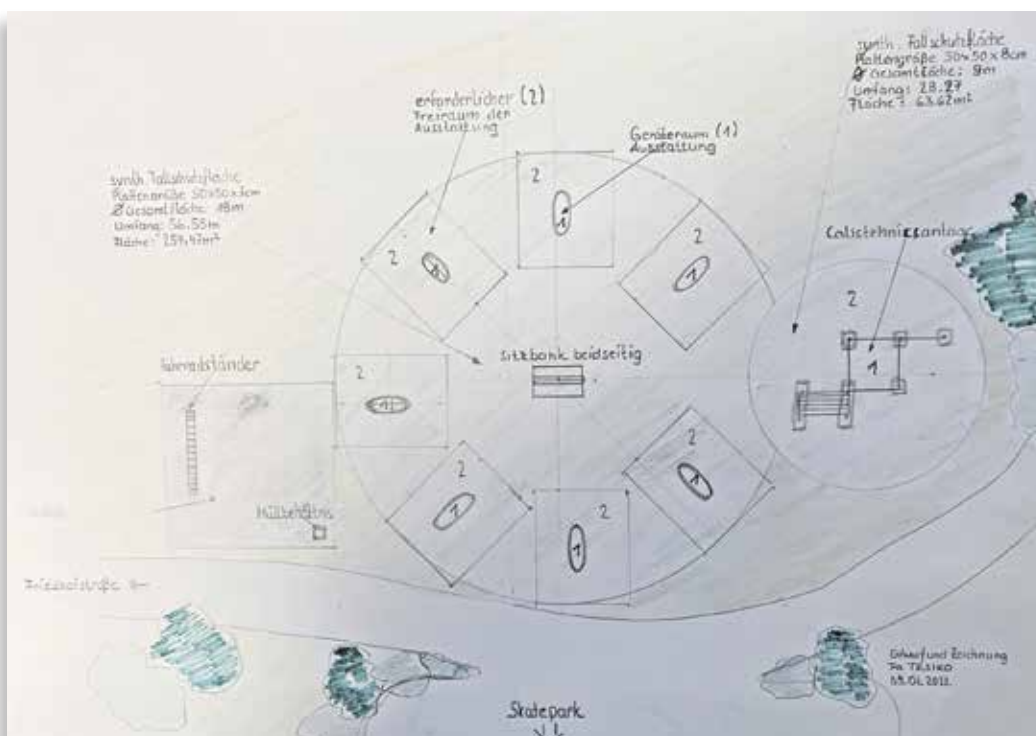
Die Skizze zeigt wie die neue Fitnessanlage aufgebaut werden könnte. (Änderungen vorbehalten/Erstskizze)
